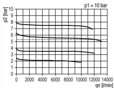
Durchflussdiagramm
