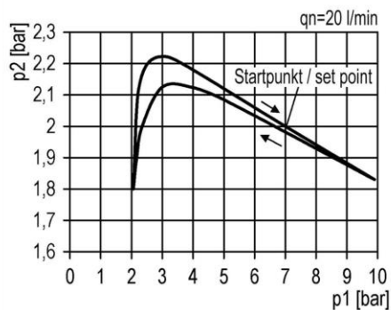
Hysteresese
